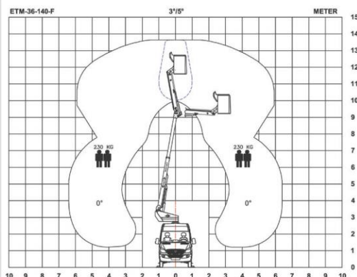
Bočný dosah so zaťažením koša 230 kg 0°
