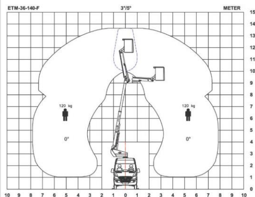
Bočný dosah so zaťažením koša 120 kg 0°
